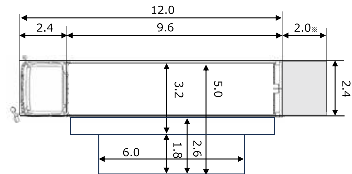
正面図 標準タイプ
